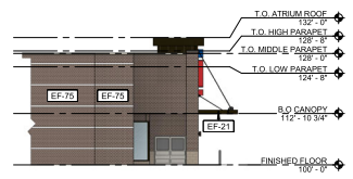
A4 SOUTH ELEVATION SCALE: 1/16" = 1'-0"
