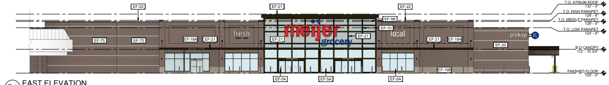
D1 EAST ELEVATION SCALE: 1/16" = 1'-0"
