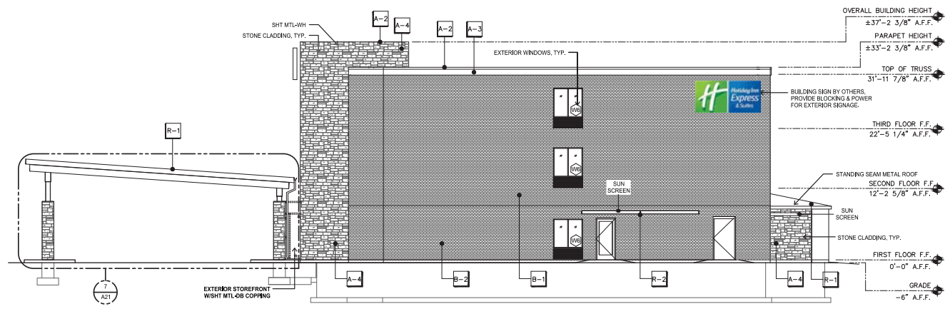
EAST ELEVATION Scale: 1/8" = 1'-0"
