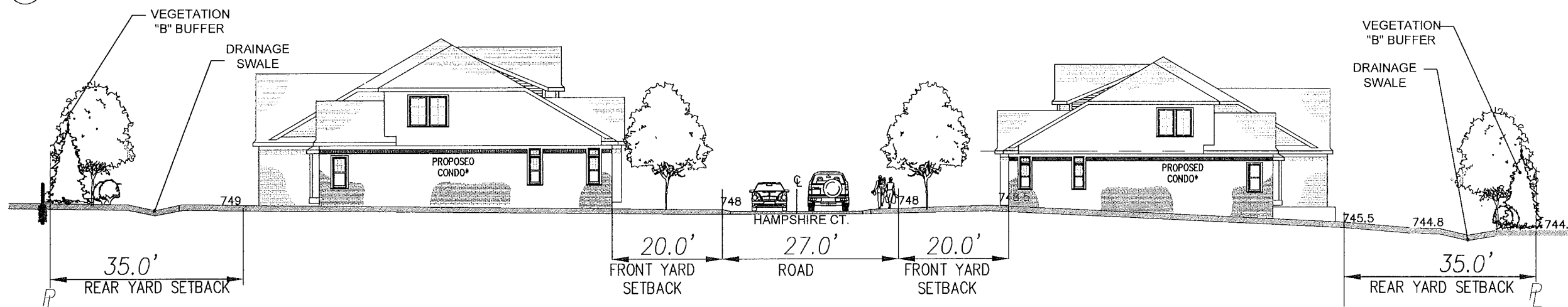
4 SECTION A-A LA-12 SCALE: 1" = 10'-0"
