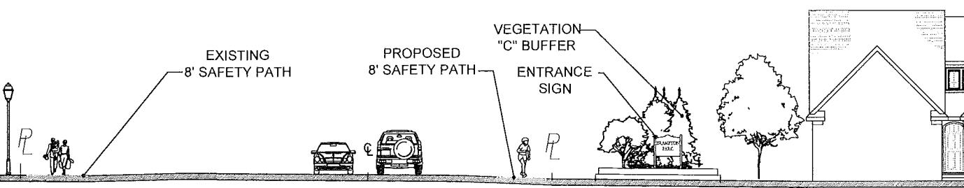
5 SECTION B-B LA-12 SCALE: 1" = 10'-0"
